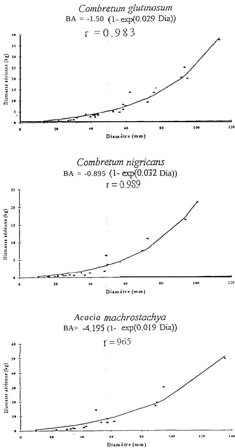
Figure 1.2 : Tarifs de biomasse sèche (bois) pour les espèces Combretum glufinosum , Combrefum nigricans et Acacia macrostachya
