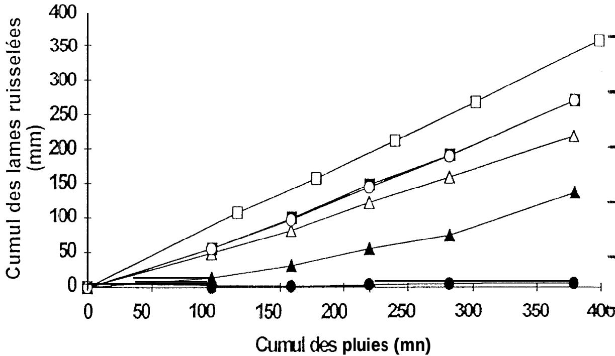
Figure 4.7: Cumul des lames ruisselées en fonction du cumul des pluies simulées sur les parcelles protégées (marques noires) et non protégées (marques transparentes), pour les couples 1 (■), 2 (●) et 3 (◻).
