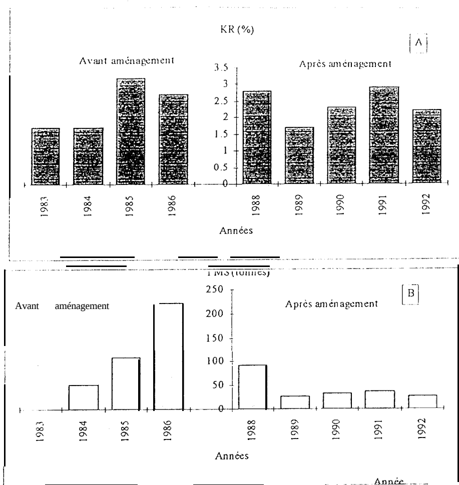
Figure 5.3. : Effets des aménagements sur le ruissellement (A) et les transports solides (5) à l'échelle du bassin versant de Keur Dianko
