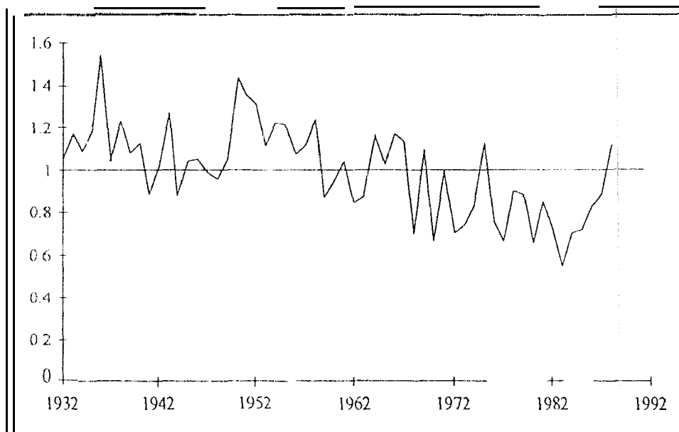
Figure 2.2 : Variation des indices pluviométriques annuels du vecteur régional (station du PAPM, Sonkorong à 30 kilomètres de Nioro du Rip)
